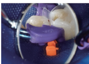
ツインリング把持脚のV字型の溝とダイヤモンドウェッジの頂点を合わせた位置で装着。
