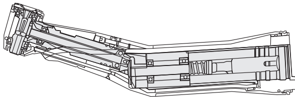
※5倍速ストレートギアードハンドピースの内部構造(例) グレーの部分全てにオイルをいきわたらせる必要があります。
