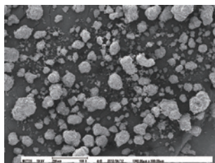
SEM像（x100）
